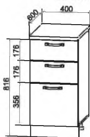
СМЯ 400 400/816/600
