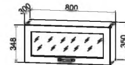
ПГС 800 800/350/300
