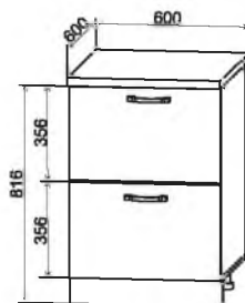
СКБ 600 600/816/600
