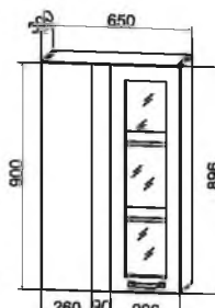
ВПУС 650 650/900/300
