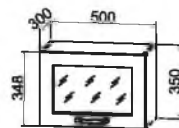
ПГС 500 500/350/300
