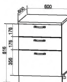
СМЯ 600 600/816/600
