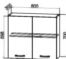
П 800 800/700/300
