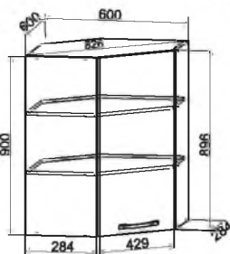
ВПУ 600 600/900/600
