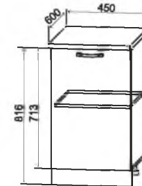
С 450 450/816/600
