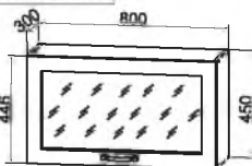
ВПГС 800 800/450/300
