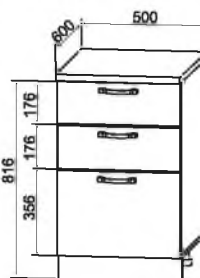
СМЯ 500 500/816/600
