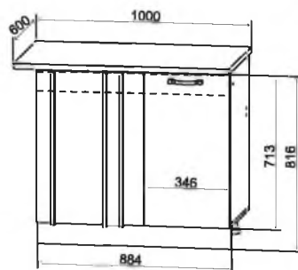
СУ 1000 1000/816/600
