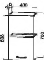
П 400 400/700/300
