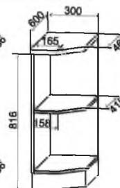
СТУ 300 300/816/600
