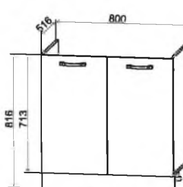
СМ 800 800/816/516
