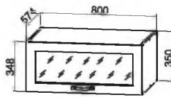
ГПГС 800 800/350/574
