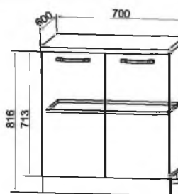
С 700 700/816/600
