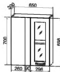
ПУС 650 650/700/300
