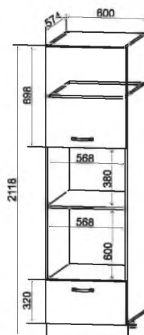
ПНС 600 600/2118/574
