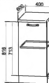
С 400 400/816/600
