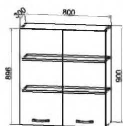
ВП 800 800/900/300
