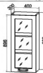
ВПС 400 400/900/300
