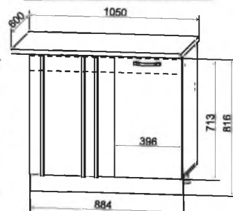
СУ 1050 1050/816/600
