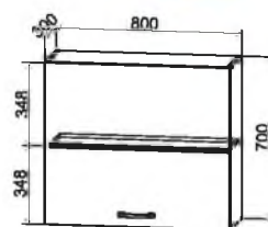
ПГПМ 800 800/700/300
