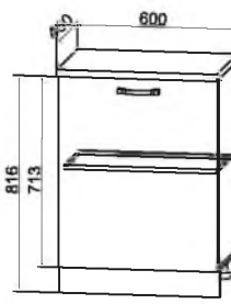
MC 600 600/816/450 Вариант 2 фасад С/СМ 601
