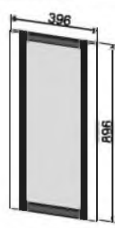
ВПВС 400 896/396 (фасад)
