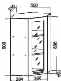
ВПУС 550 550/900/550
