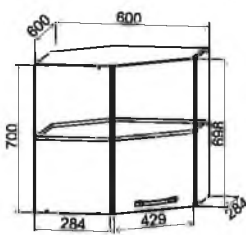
ПУ 600 600/700/600
