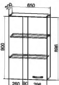
ВПУ 650 650/900/300
