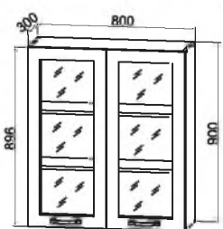
ВПС 800 800/900/300
