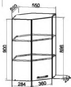
ВПУ 550 550/900/550
