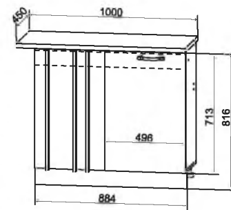
МСУ 1000 1000/816/450
